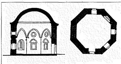
İdris Baba Türbesi ile türbenin kesiti ve planı - Peçuy / Macaristan
